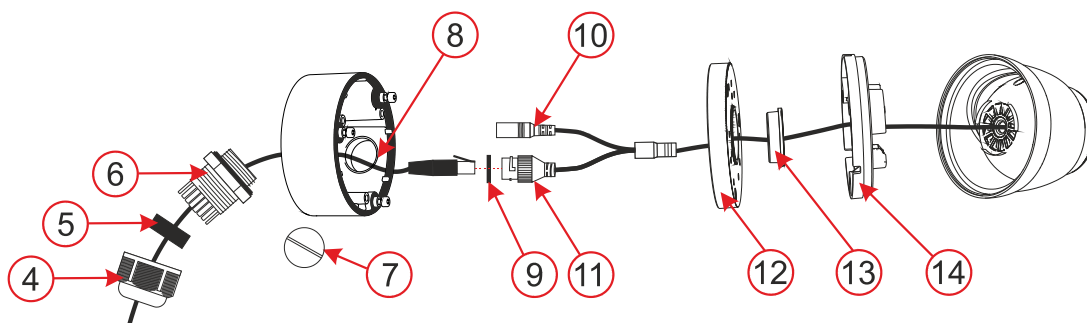
Obrázek 3: Postup instalace s použitím montážní patice
