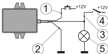
Příklad zapojení ve vozidle: 1 - červený; 2 - černý; 3 - bílý; 4 - světelná houkačka; 5 - dálková světlá
