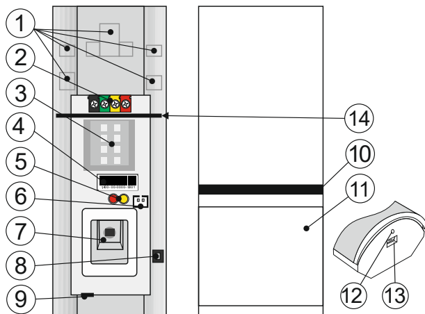
Obrázek 1: 1 – vytlamovací otvory pro kabeláž; 2 – svorky sběrnice; 3 – MW senzor; 4 – sériové číslo; 5 – signálky pro indikaci stavů; 6 – konektor pro připojení sabotážního spínače kloubového držáku JA-191PL; 7 – PIR senzor; 8 – sabotážní spínač; 9 – západka elektroniky; 10 – světlodod; 11 – čočka PIR detektoru; 12 – otvor pro aretační šroub; 13 – západka krytu; 14 – přepážka pro ochranu MW senzoru od vodičů
