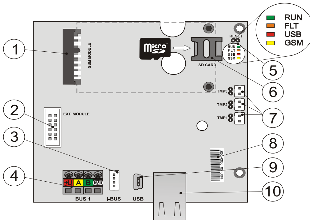
1 - konektor pro GSM komunikátor; 2 – konektor pro přidavné moduly; 3 - konektor sběrnice pro interní radiový modul JA-11xR; 4 - svorkovnice sběrnice; 5 - signály s propojkou RESET; 6 držák micro SD karty; 7 - konektory sabotážních spínačů skříně; 8 – seriové číslo; 9 - miniUSB konektor; 10 - konektor LAN
