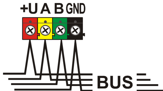
Svorkovnice sběrnice
