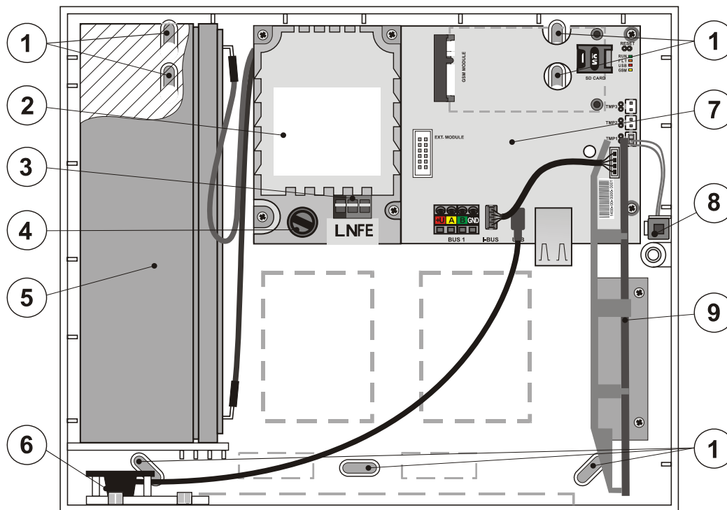
1 - otvory pro montáž skříně na zed; 2 – modul zdroje; 3 - svorkovnice síťového přívodu; 4 – síťová pojistka; 5 - záložní akumulátor; 6 - USB konektor pro připojení k PC; 7 - deska ústředny; 8 – sabotážní spínač skříně; 9 - držák pro radiový modul JA-11xR
